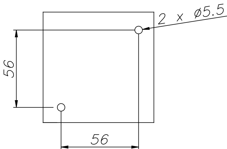
PLANTILLA DE INSTALACIÓN INSTALLATION TEMPLATE
